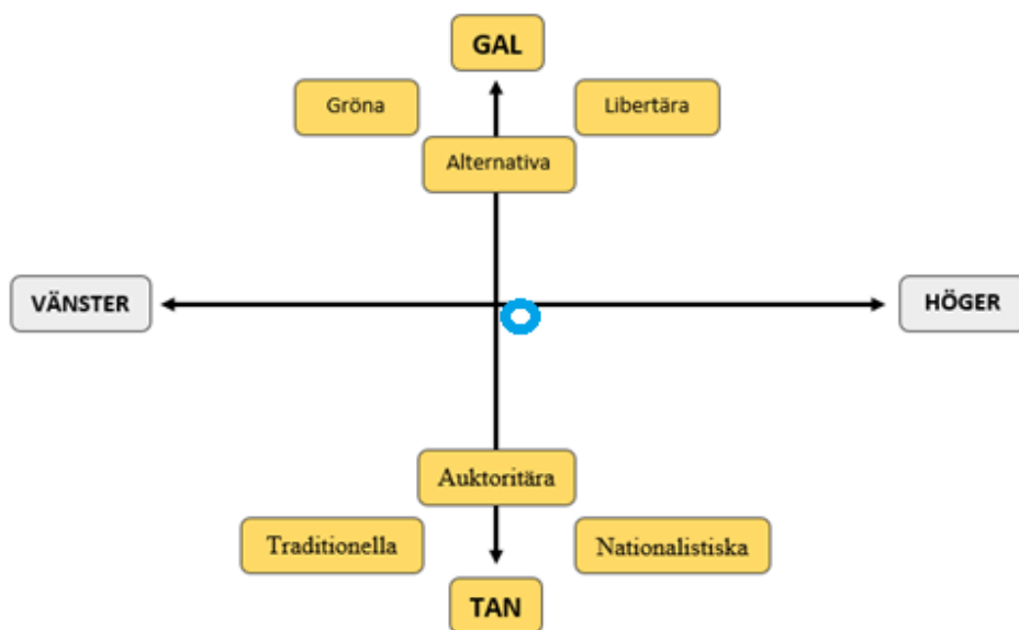
Diagram 5.4.1 Var Sverigedemokraterna kan placeras idag på den två dimensionella skalan.
