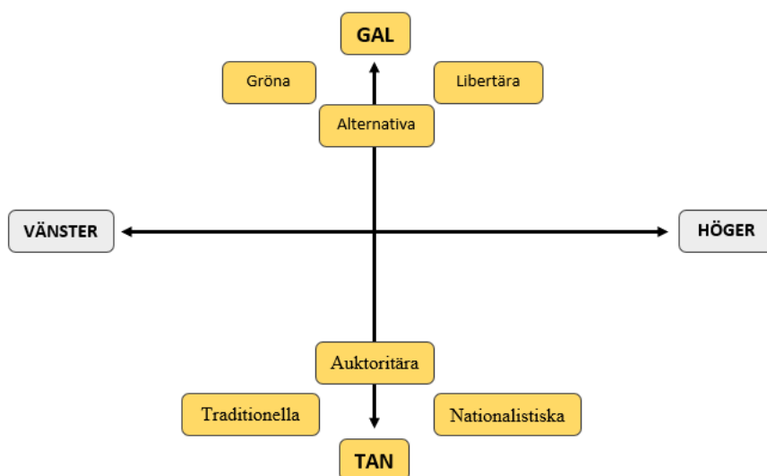
Diagram 3.4.1 GAL-TAN på den tvådimensionella skalan. Bearbetat efter en okänd källa från Twitter.
