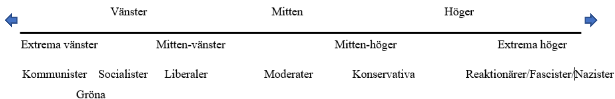
Diagram 3.3.1. Vänster-högerskalan inom den moderna världen. Bearbetat efter Woshinsky (2008, 112).
